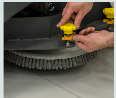
Eenvoudig onderhoud: nieuwe onderhoudsvrije motor, hoogwaardige aandrijving en geel gemarkeerde afstelpunten.
